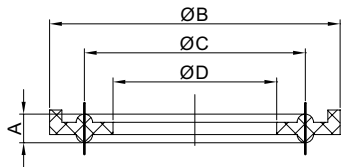
卡箍垫圈 Gasket for ferrule
