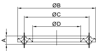
卡箍垫圈 Gasket for ferrule
