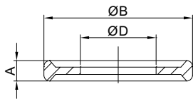
卡箍垫圈 Gasket for ferrule
